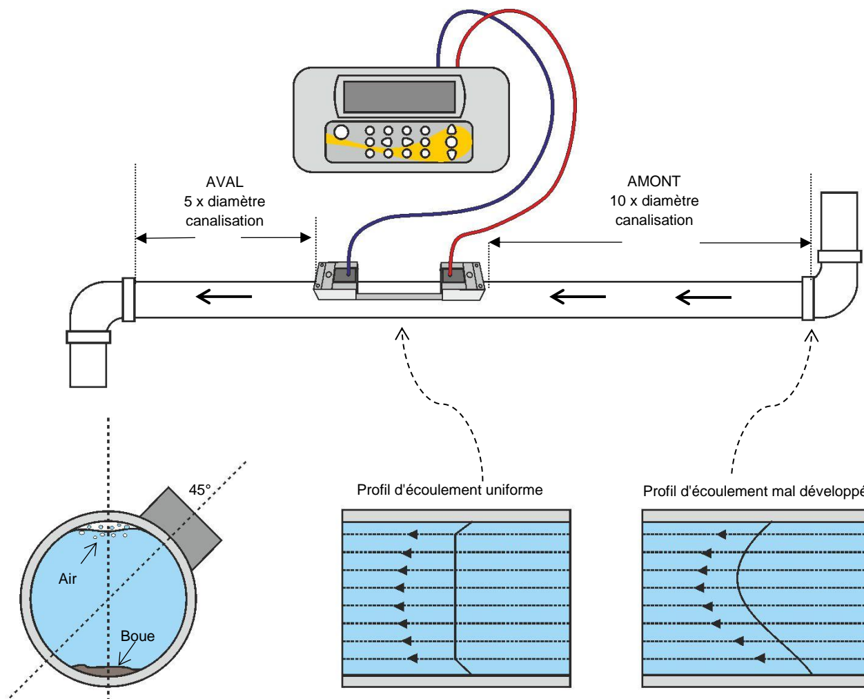
Figure 8 Emplacement de l'appareil
