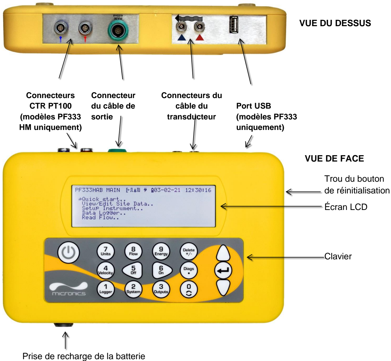
Figure 5 Appareil Portaflow (modèle PF333HM représenté sur l'illustration)
