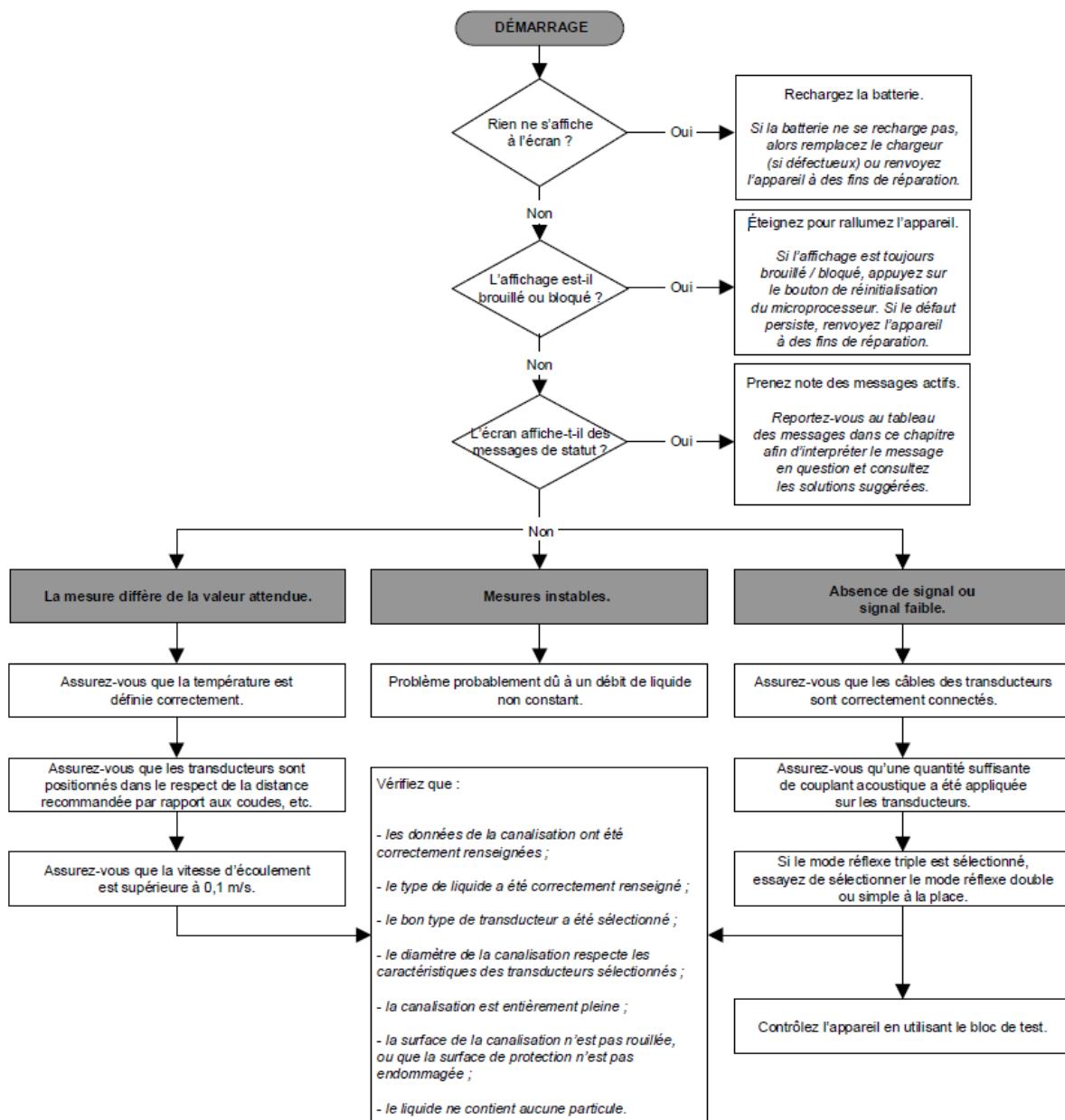
Figure 16 Diagramme de dépannage
