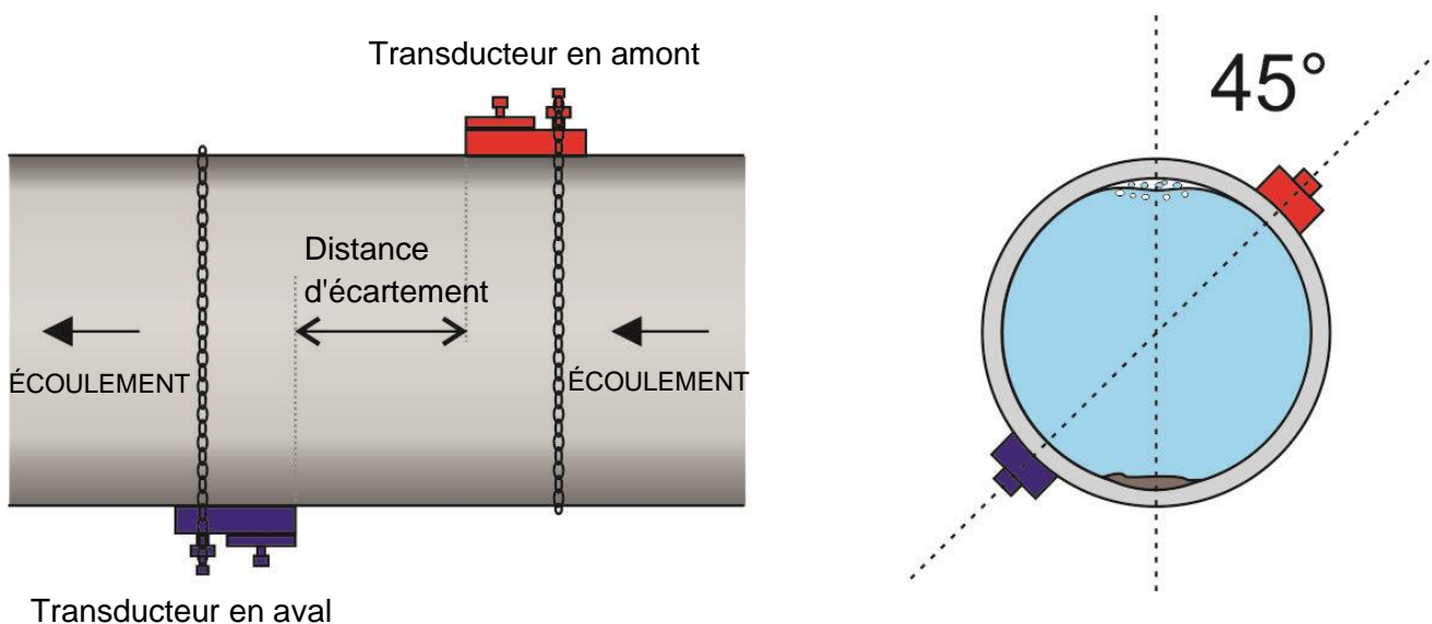
Figure 12 Positions des transducteurs pour le Mode Diagonale
