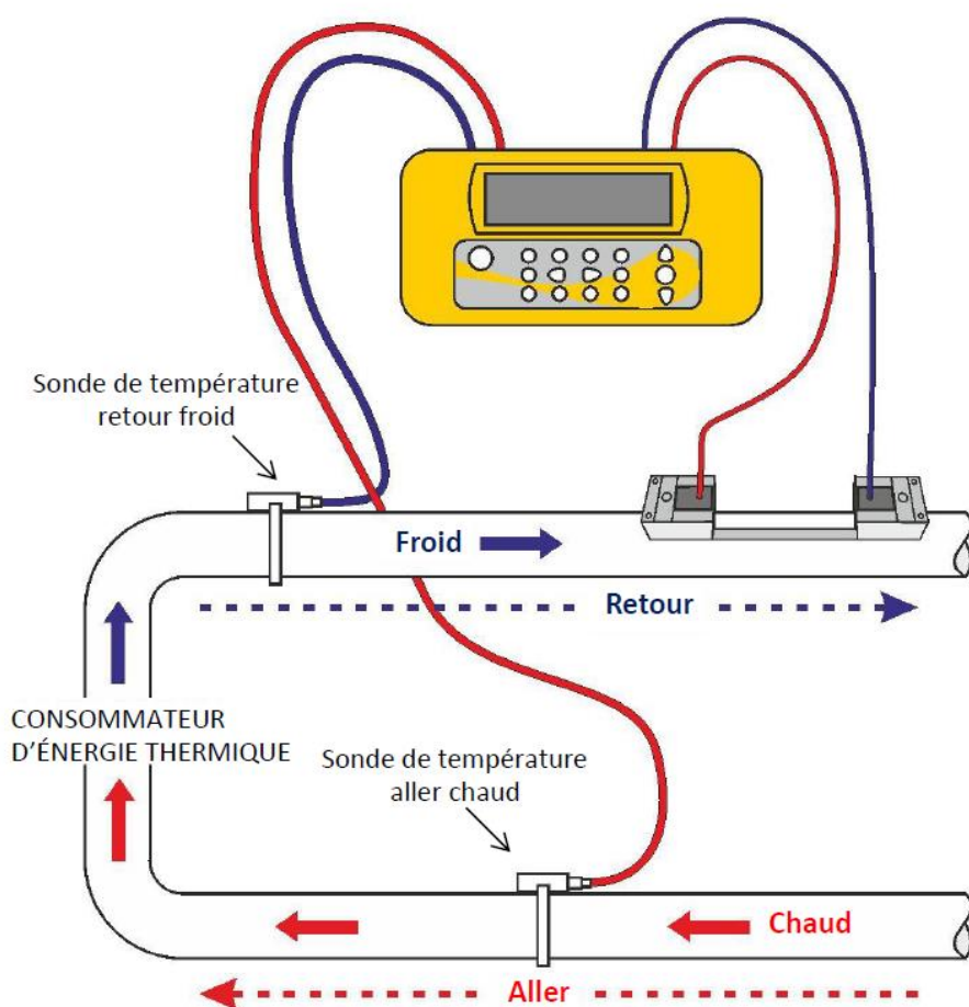
Figure 13 Positionnement du capteur de température Portaflow 333 (système de chaudière)
