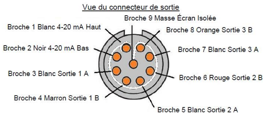
Figure 15 Câblage de sortie
