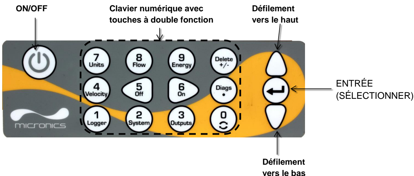
Figure 6 Clavier du Portaflow
