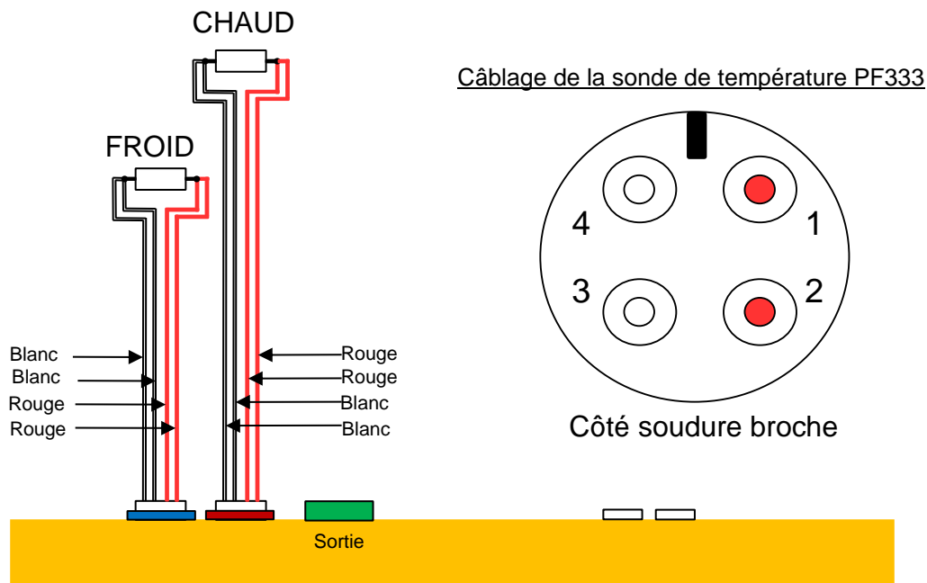
Figure 14 Câblage de la sonde de température PF333
