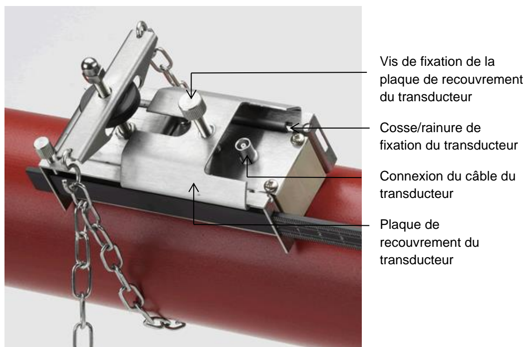
Figure 11 Transducteur dans rail de guidage
